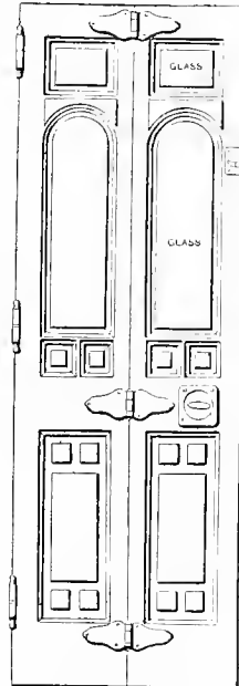
Fig. 1791. DOOR FOR GOULD VESTIBULE.
